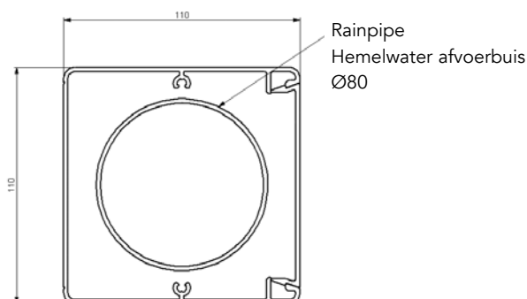
Post with drain Stander met afvoerpijp
