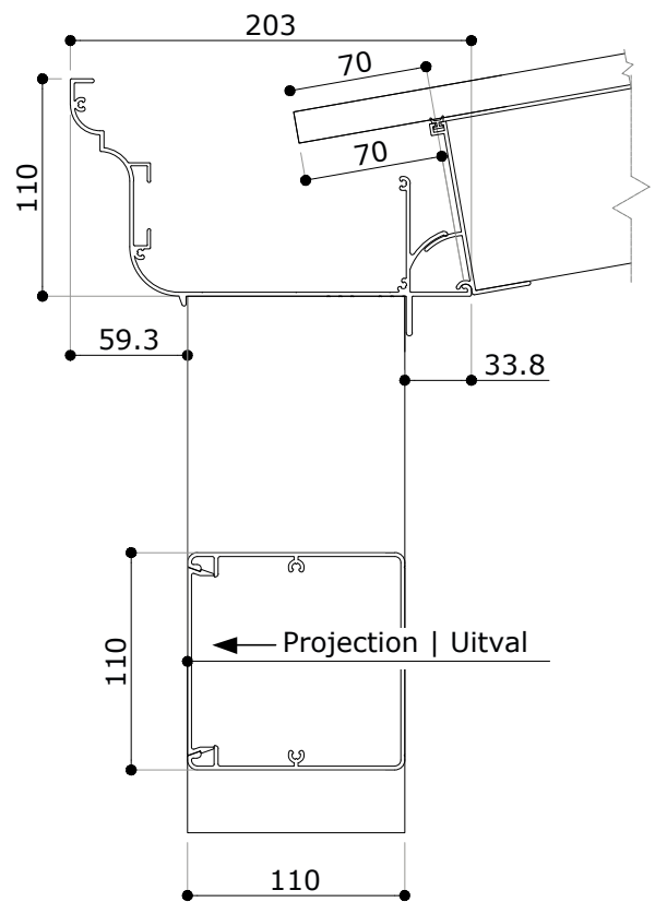
Classic gutter profile Klassiek gootprofiel
