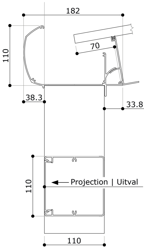
Standard gutter profil Standaard gootprofiel
