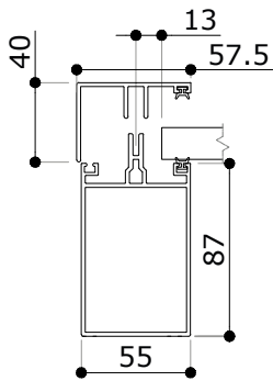
Beam with side cover profile Ligger met eindlijst
