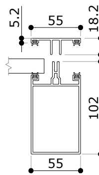
Beam with cover profile Ligger met afdekljst
