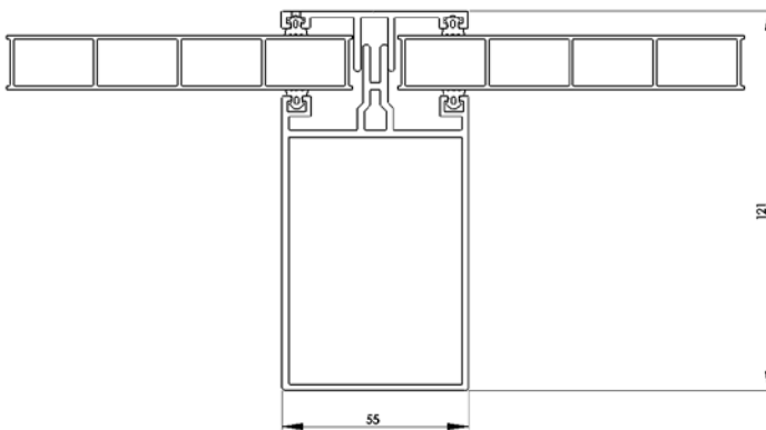
Beam with polycarbonate sheet 16 mm Ligger met polycarbonaat plaat 16 mm
