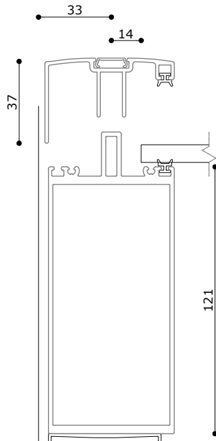
Beam with side cover profile Ligger met eindlijst
