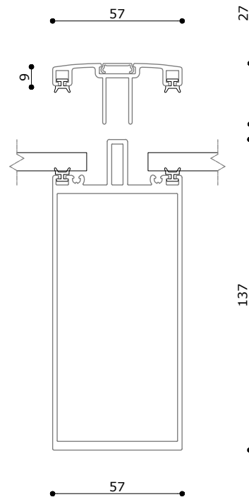
Beam with cover profile Ligger met afdekljst
